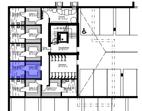
Untergeschoss
