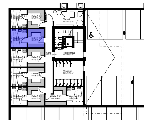
Untergeschoss
